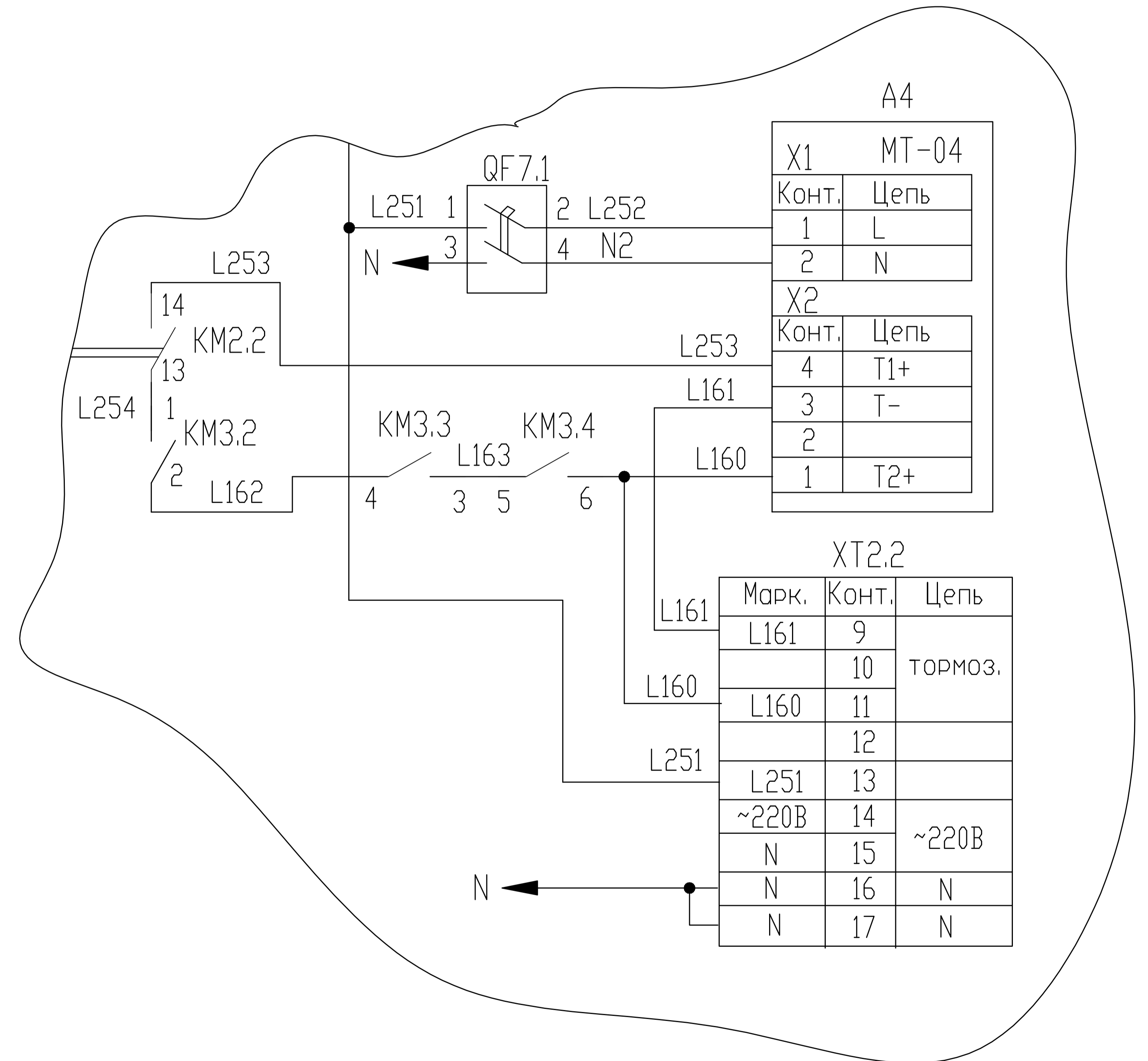
Подключение для модуля тормоза МТ-04 УИРФ.468335.004-01
